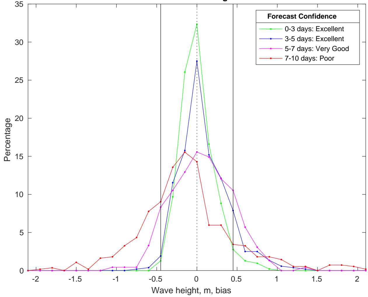
NDBC 46054 vs CMEMS Waves Bias Histogram: 13-Feb-2025
