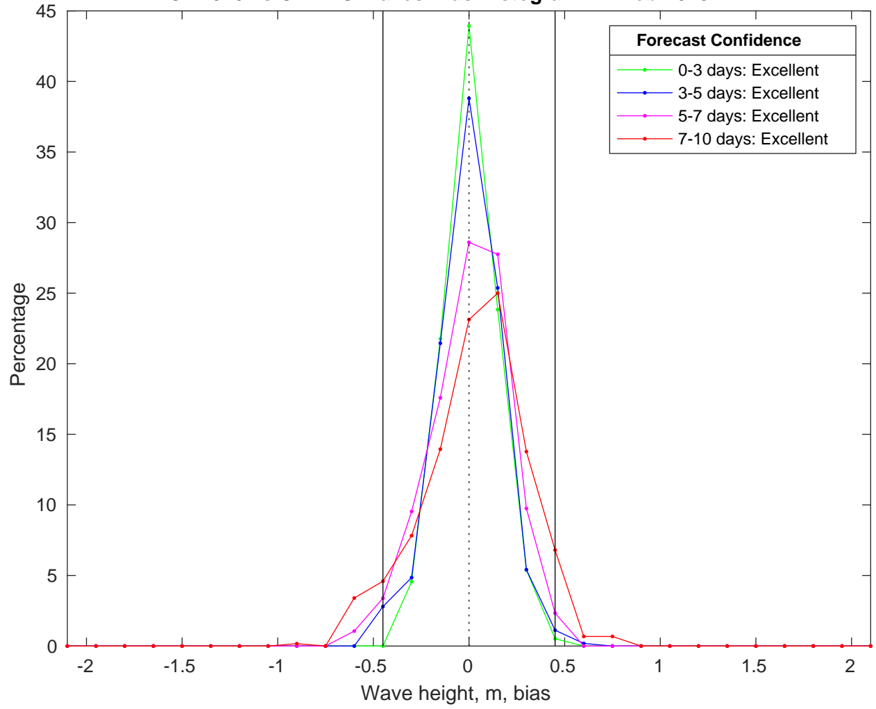
NDBC 41040 vs CMEMS Waves Bias Histogram: 14-Feb-2025
