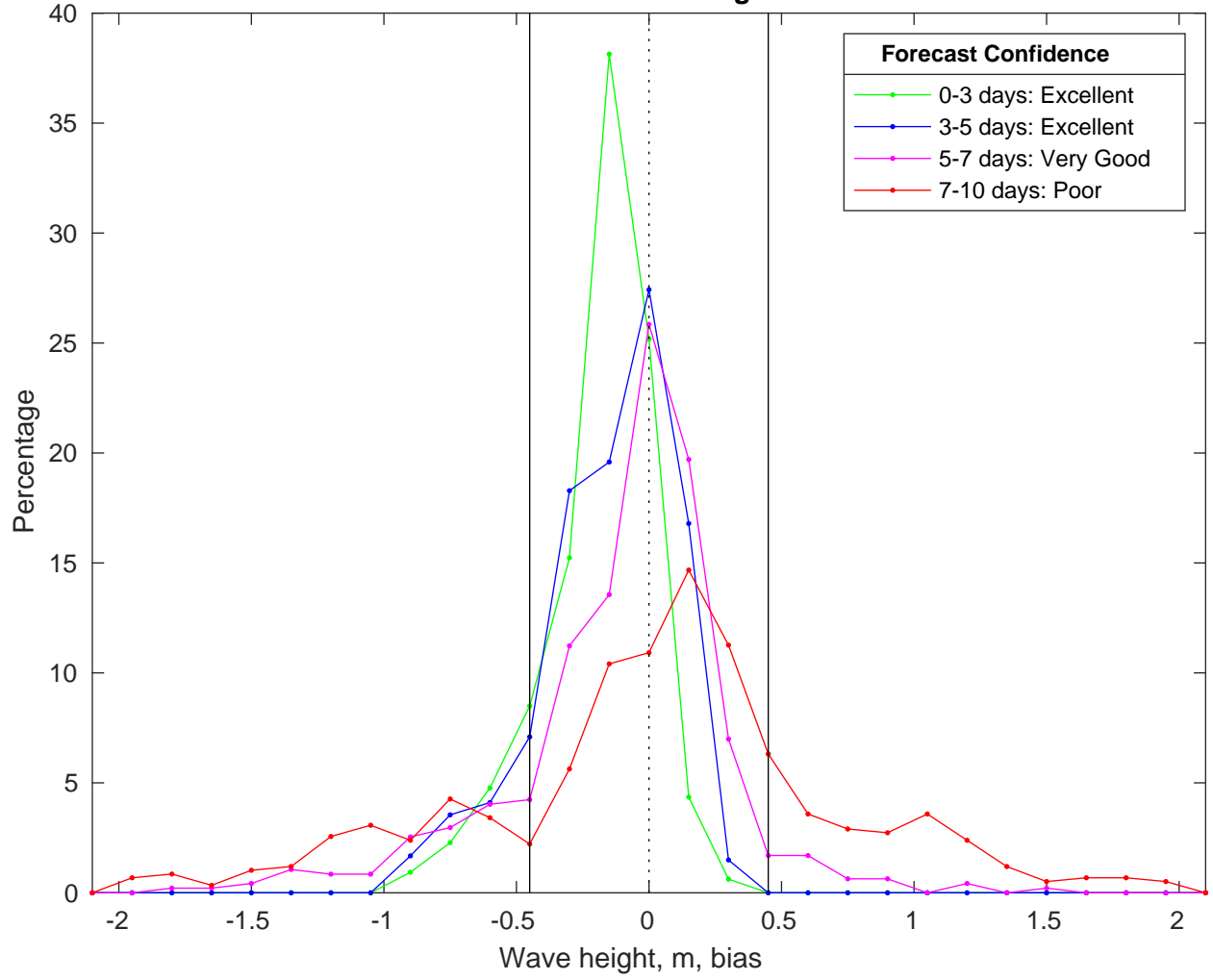
NDBC 42019 vs CMEMS Waves Bias Histogram: 14-Feb-2025
