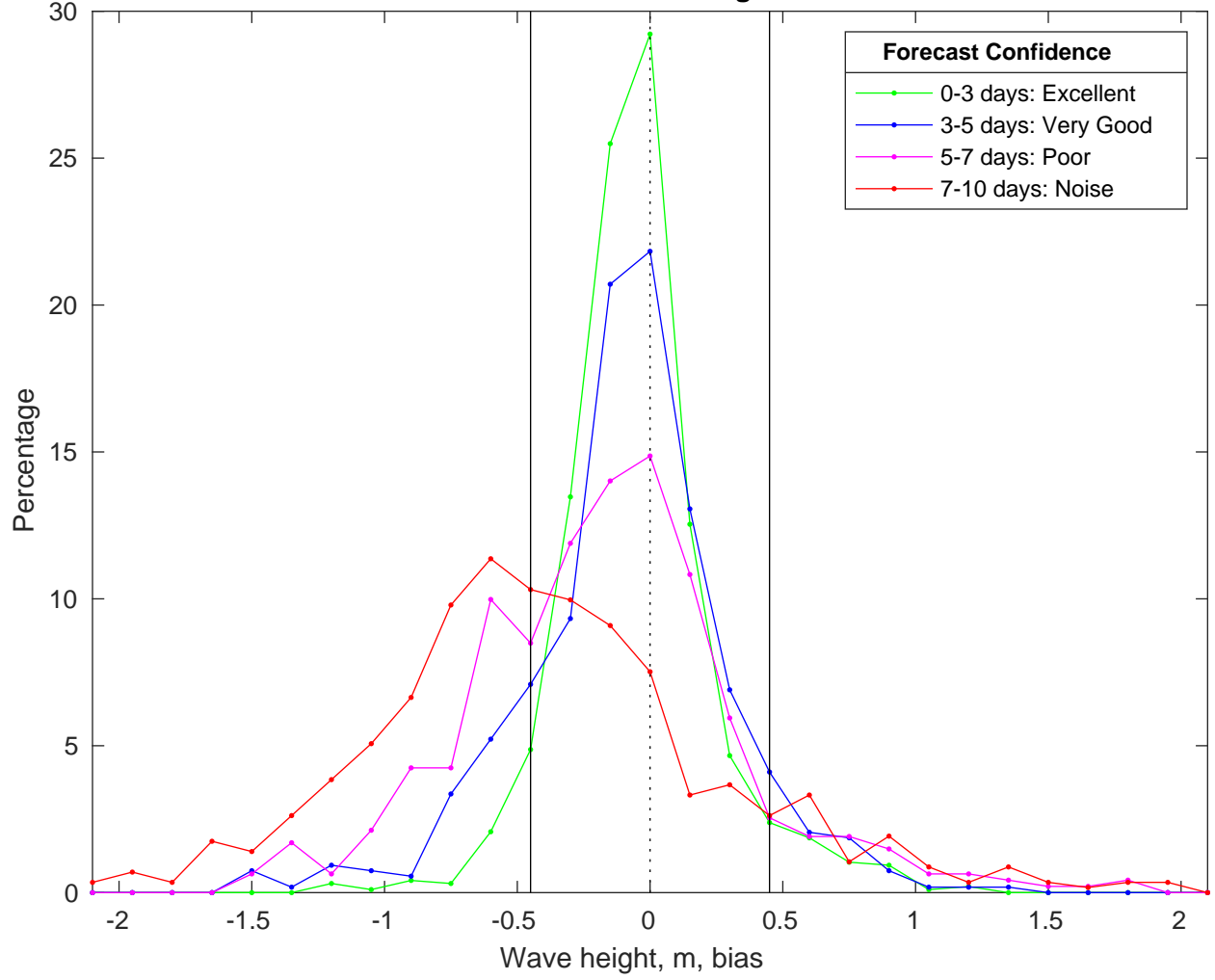
NDBC 46028 vs CMEMS Waves Bias Histogram: 14-Feb-2025
