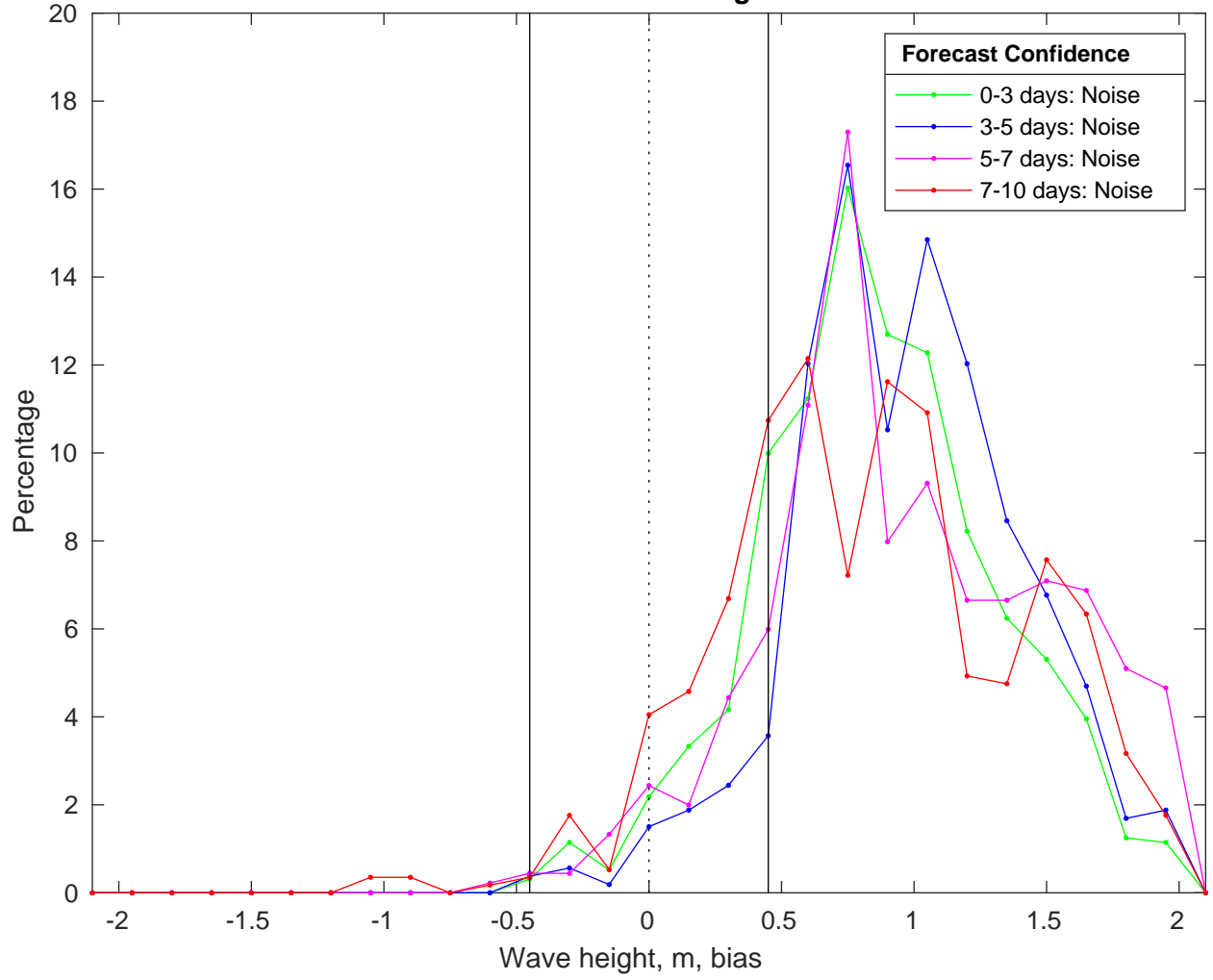
NDBC 46053 vs CMEMS Waves Bias Histogram: 14-Feb-2025
