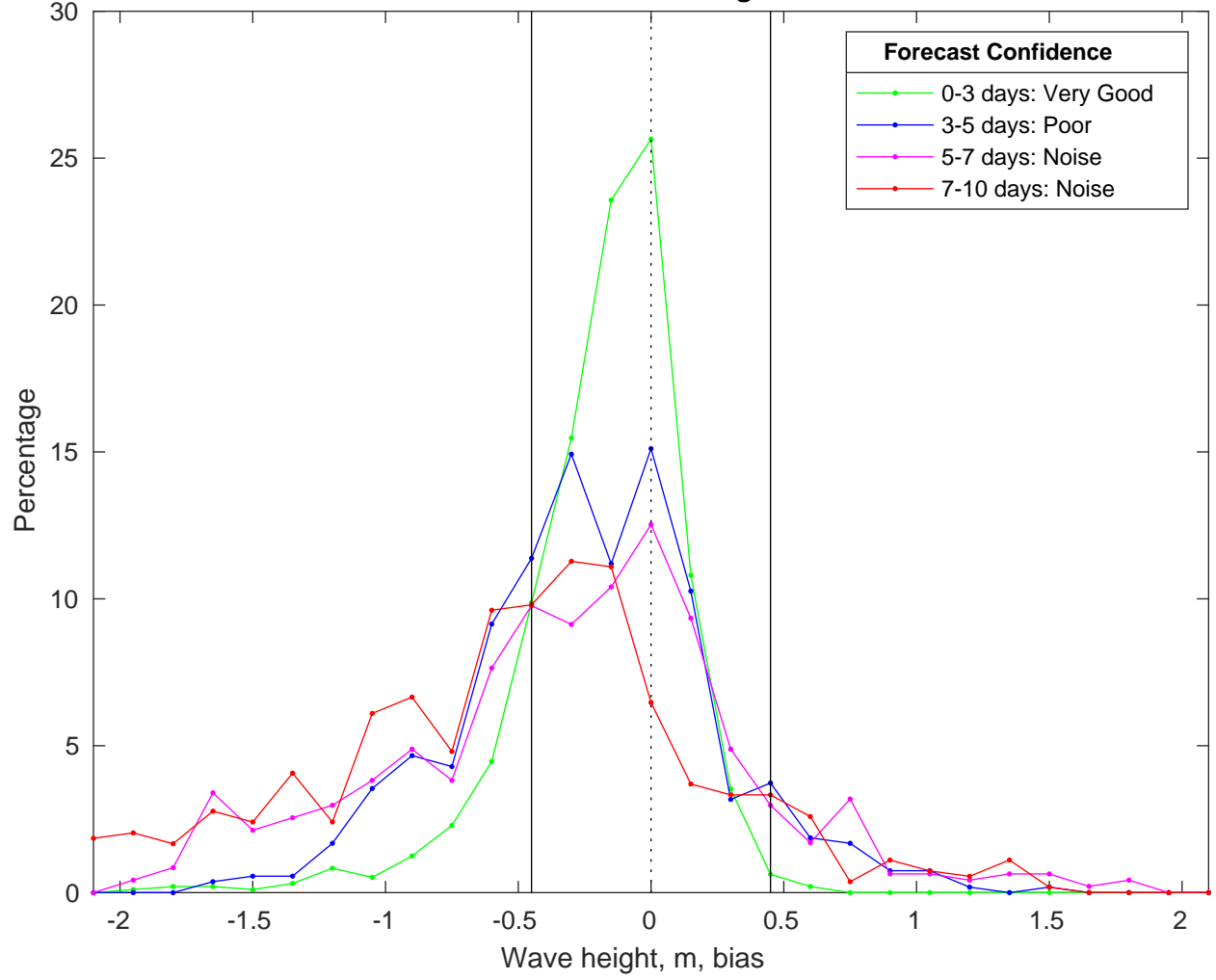
NDBC 46246 vs CMEMS Waves Bias Histogram: 14-Feb-2025
