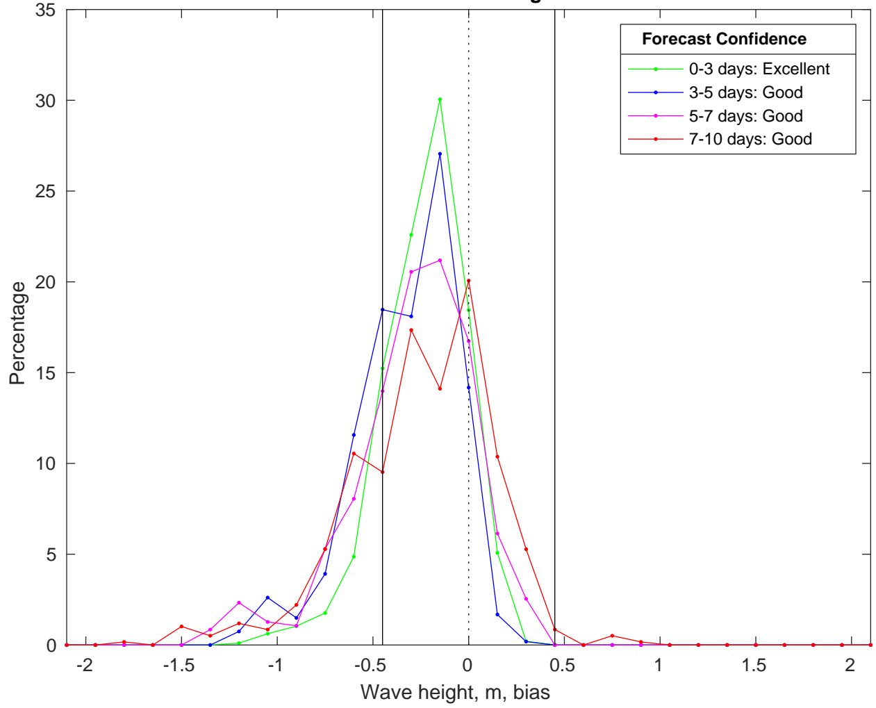
NDBC 52211 vs CMEMS Waves Bias Histogram: 14-Feb-2025
