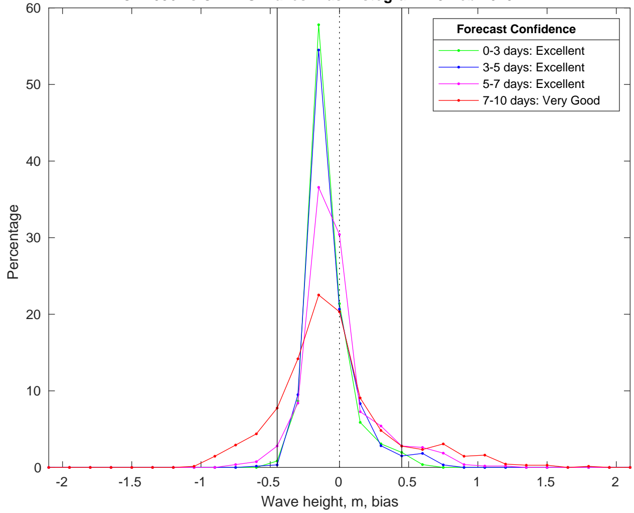
NDBC 42036 vs CMEMS Waves Bias Histogram: 19-Feb-2025
