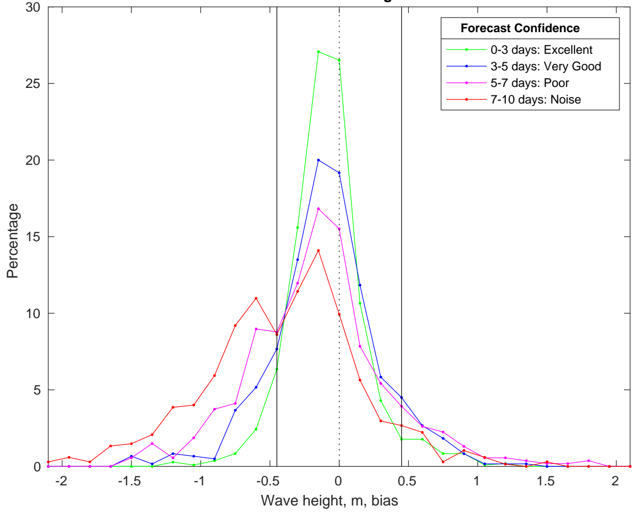
NDBC 46028 vs CMEMS Waves Bias Histogram: 19-Feb-2025
