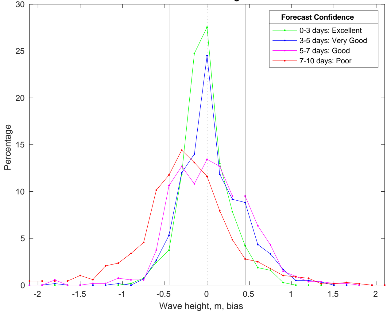
NDBC 46054 vs CMEMS Waves Bias Histogram: 19-Feb-2025
