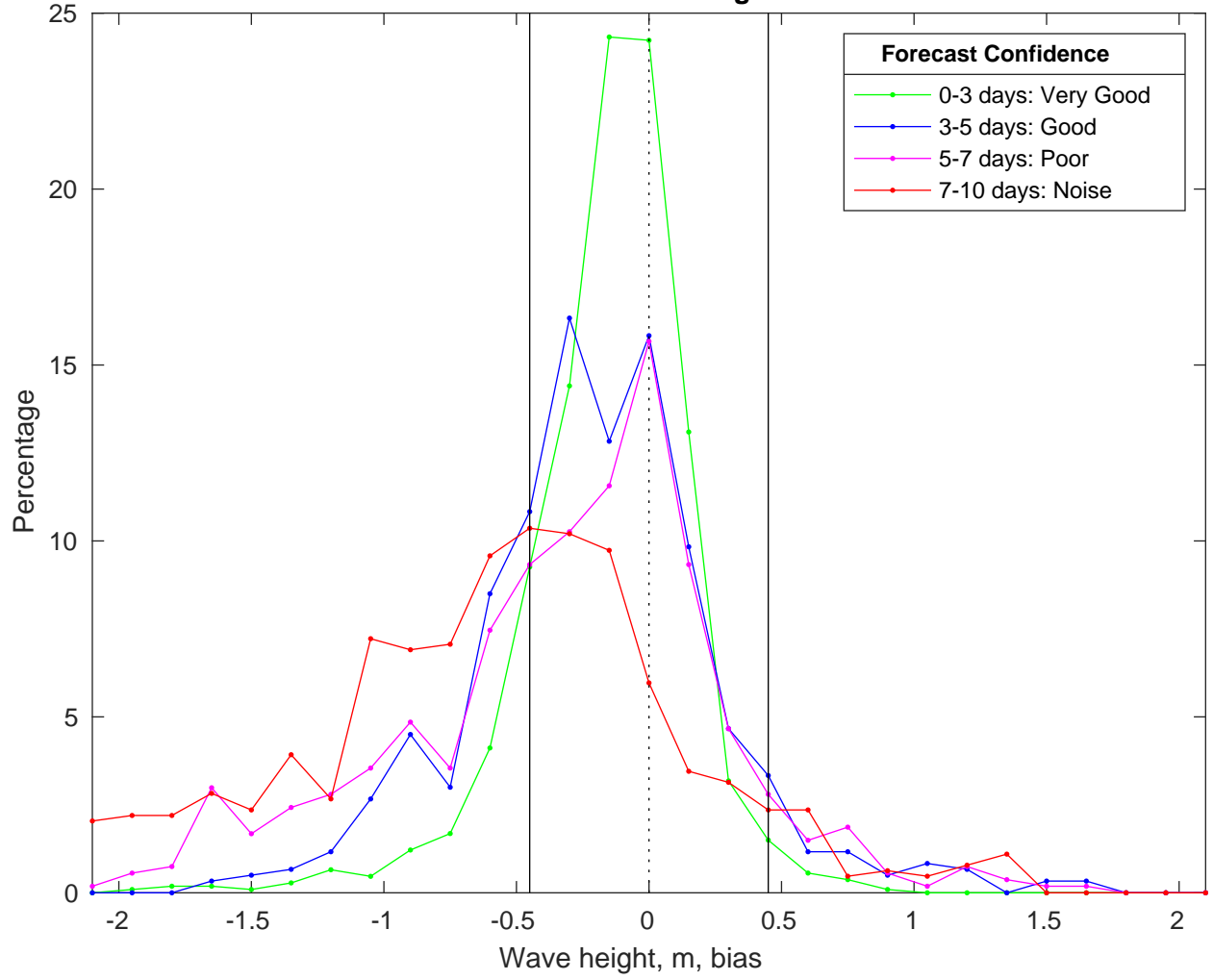
NDBC 46246 vs CMEMS Waves Bias Histogram: 19-Feb-2025
