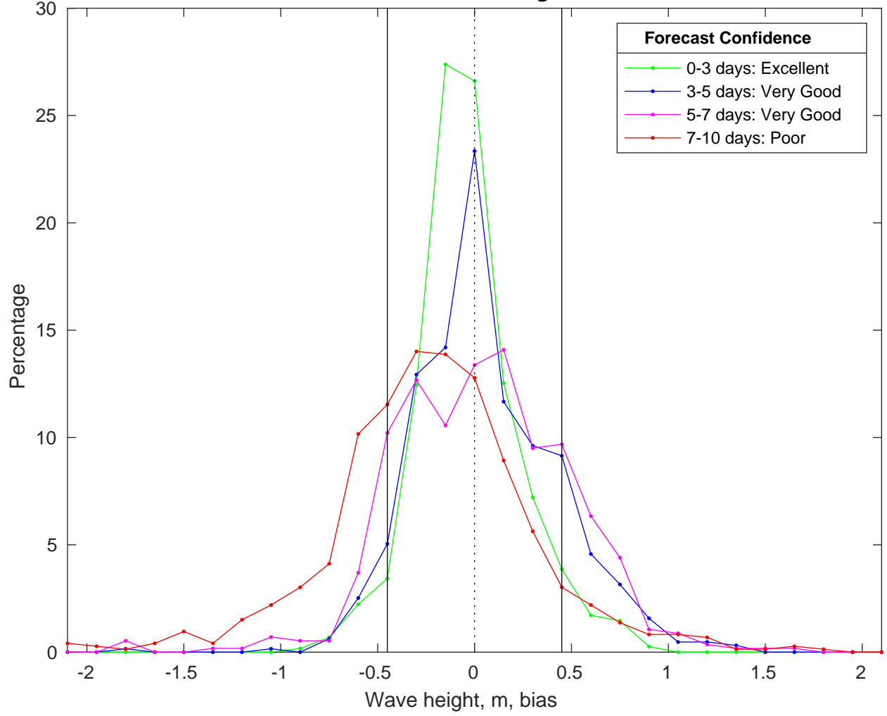
NDBC 46054 vs CMEMS Waves Bias Histogram: 21-Feb-2025
