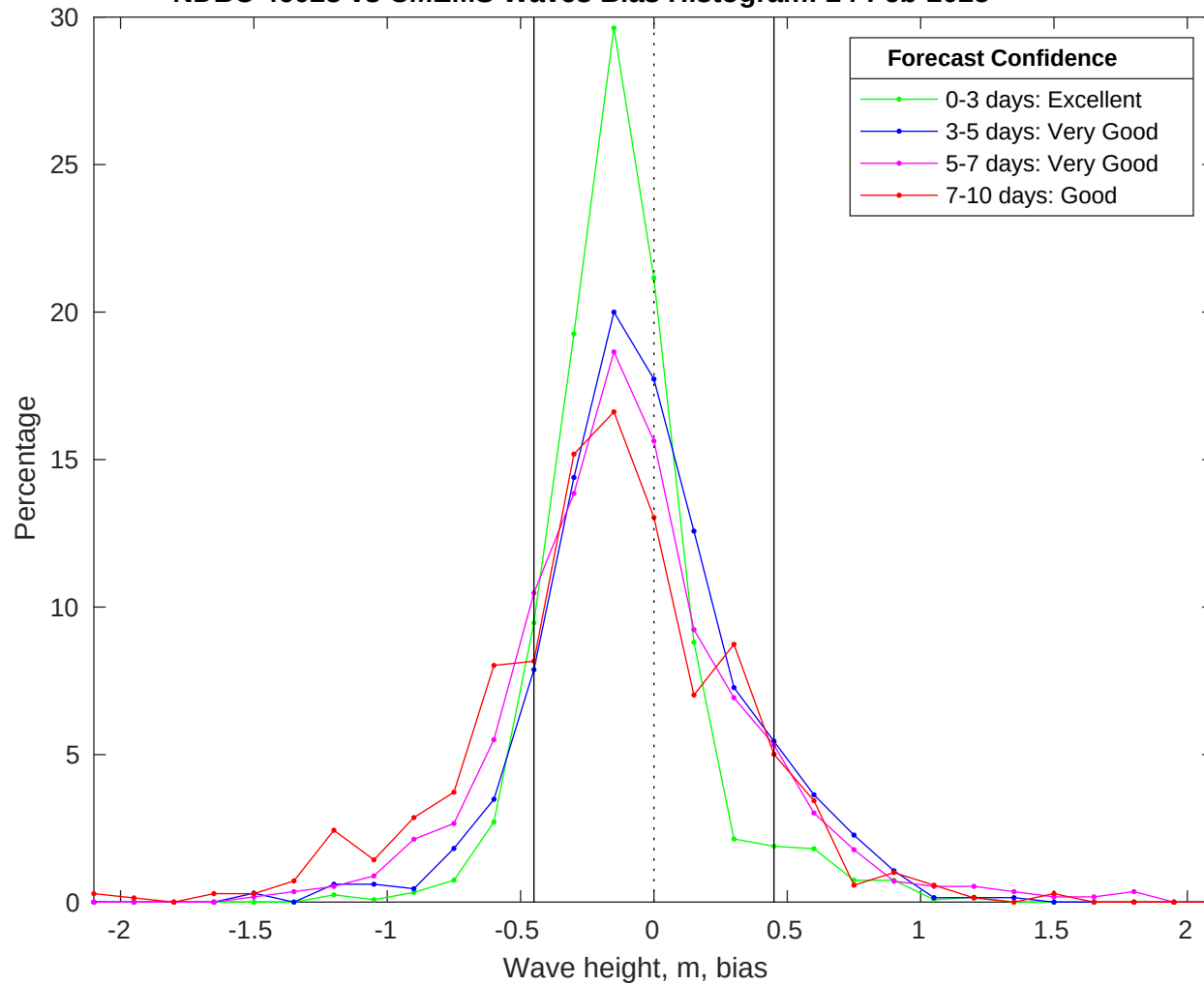
NDBC 46028 vs CMEMS Waves Bias Histogram: 24-Feb-2025
