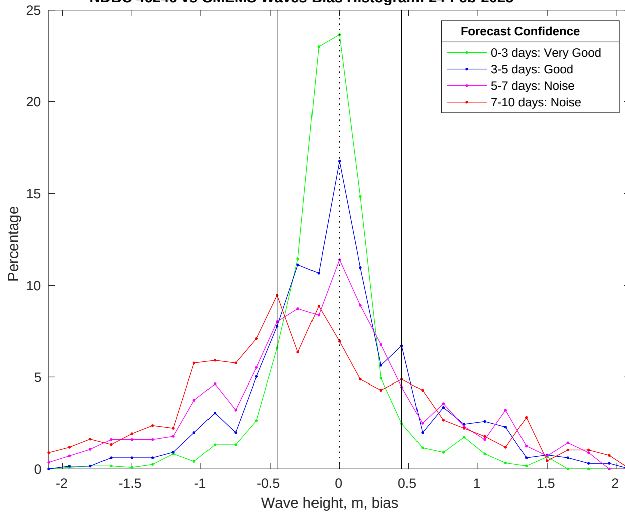
NDBC 46246 vs CMEMS Waves Bias Histogram: 24-Feb-2025
