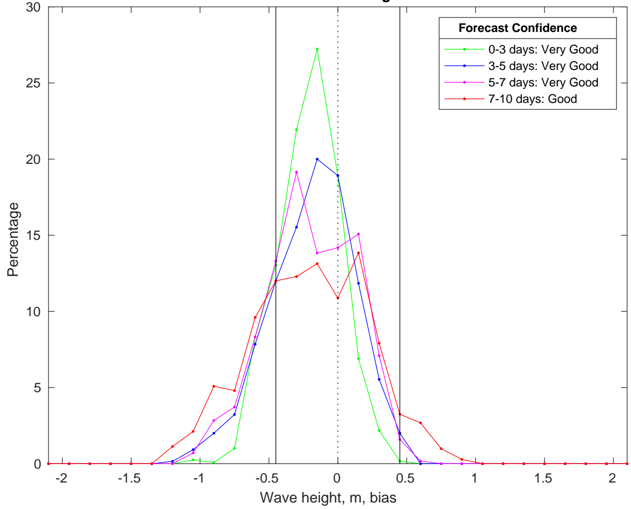
NDBC 52213 vs CMEMS Waves Bias Histogram: 24-Feb-2025
