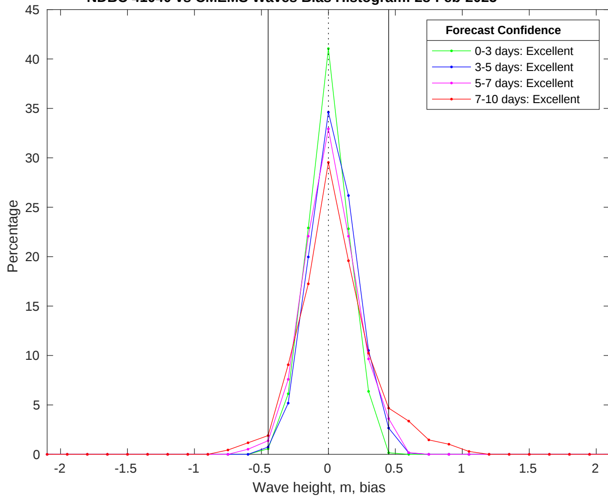
NDBC 41040 vs CMEMS Waves Bias Histogram: 28-Feb-2025
