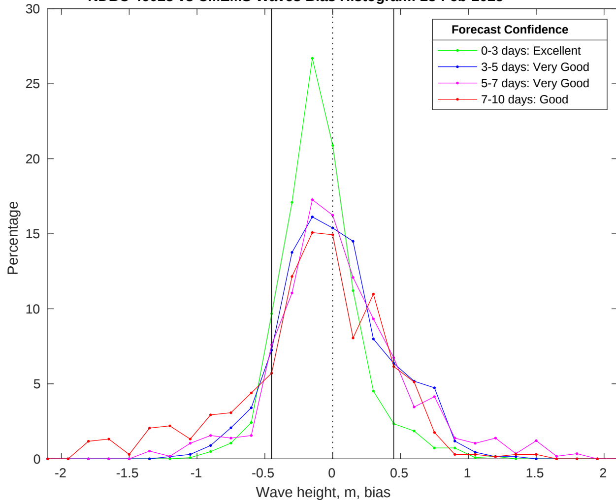
NDBC 46028 vs CMEMS Waves Bias Histogram: 28-Feb-2025
