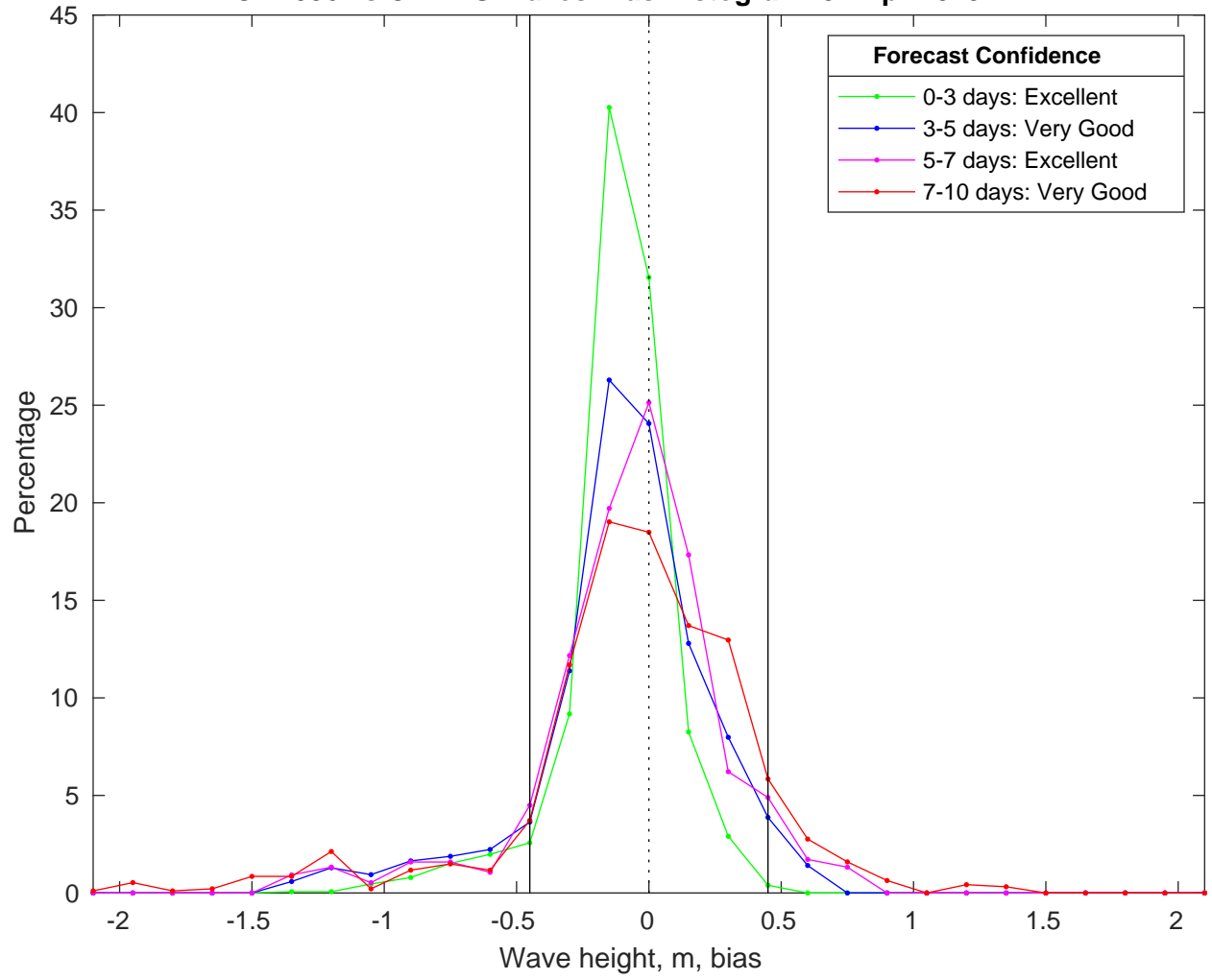
NDBC 42036 vs CMEMS Waves Bias Histogram: 02-Apr-2025
