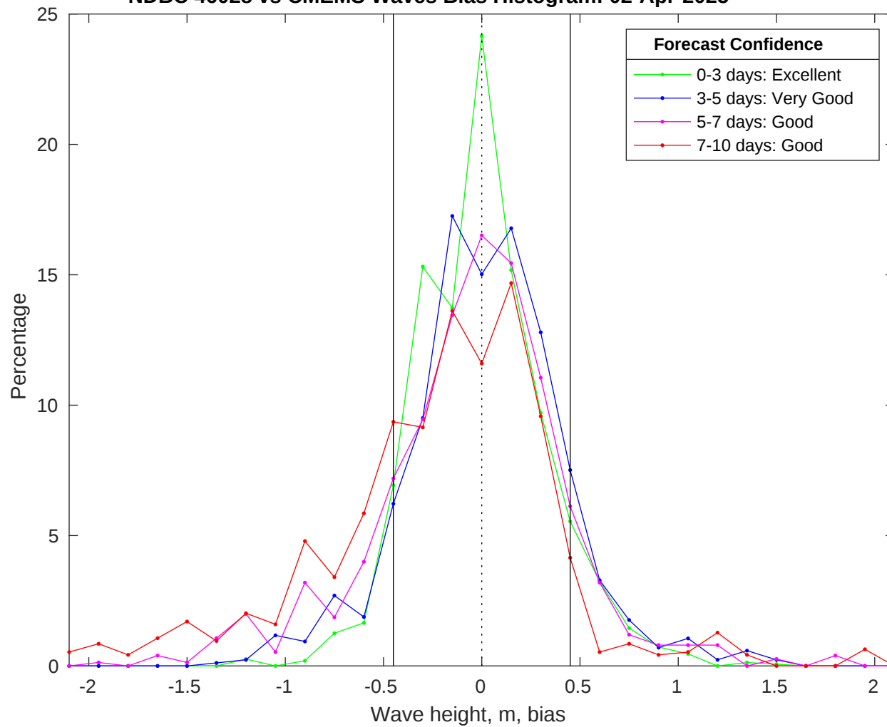
NDBC 46028 vs CMEMS Waves Bias Histogram: 02-Apr-2025
