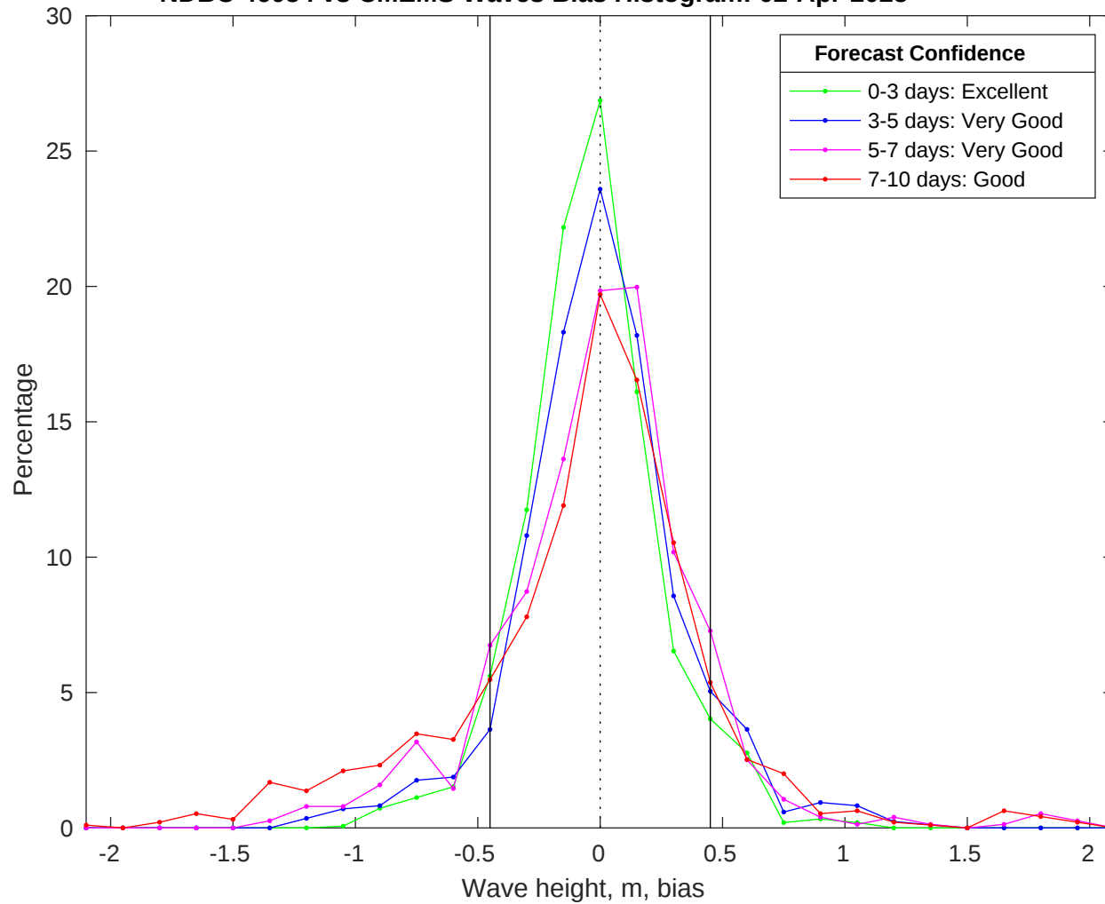
NDBC 46054 vs CMEMS Waves Bias Histogram: 02-Apr-2025
