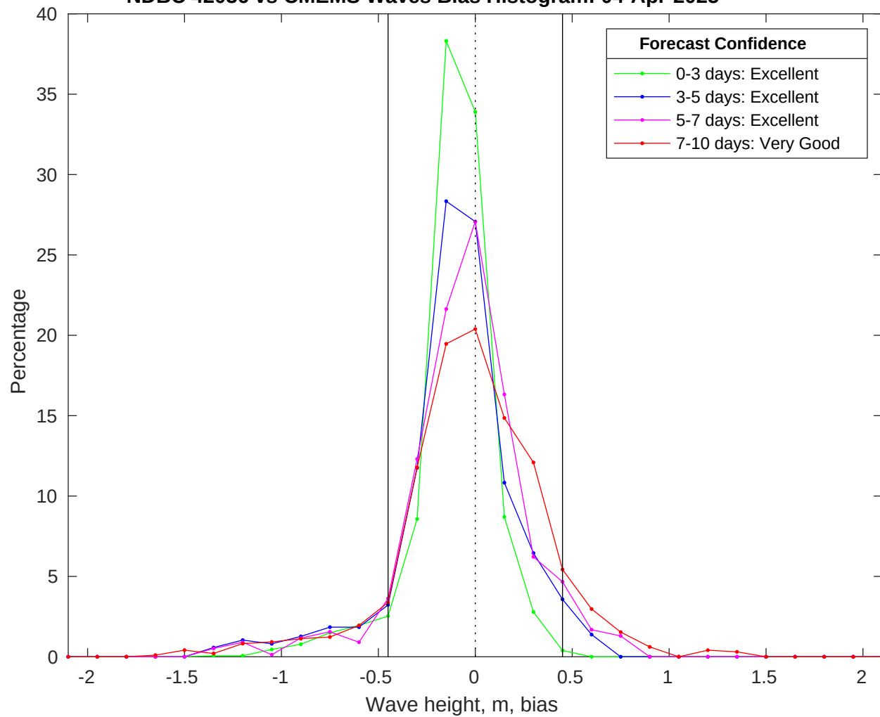
NDBC 42036 vs CMEMS Waves Bias Histogram: 04-Apr-2025
