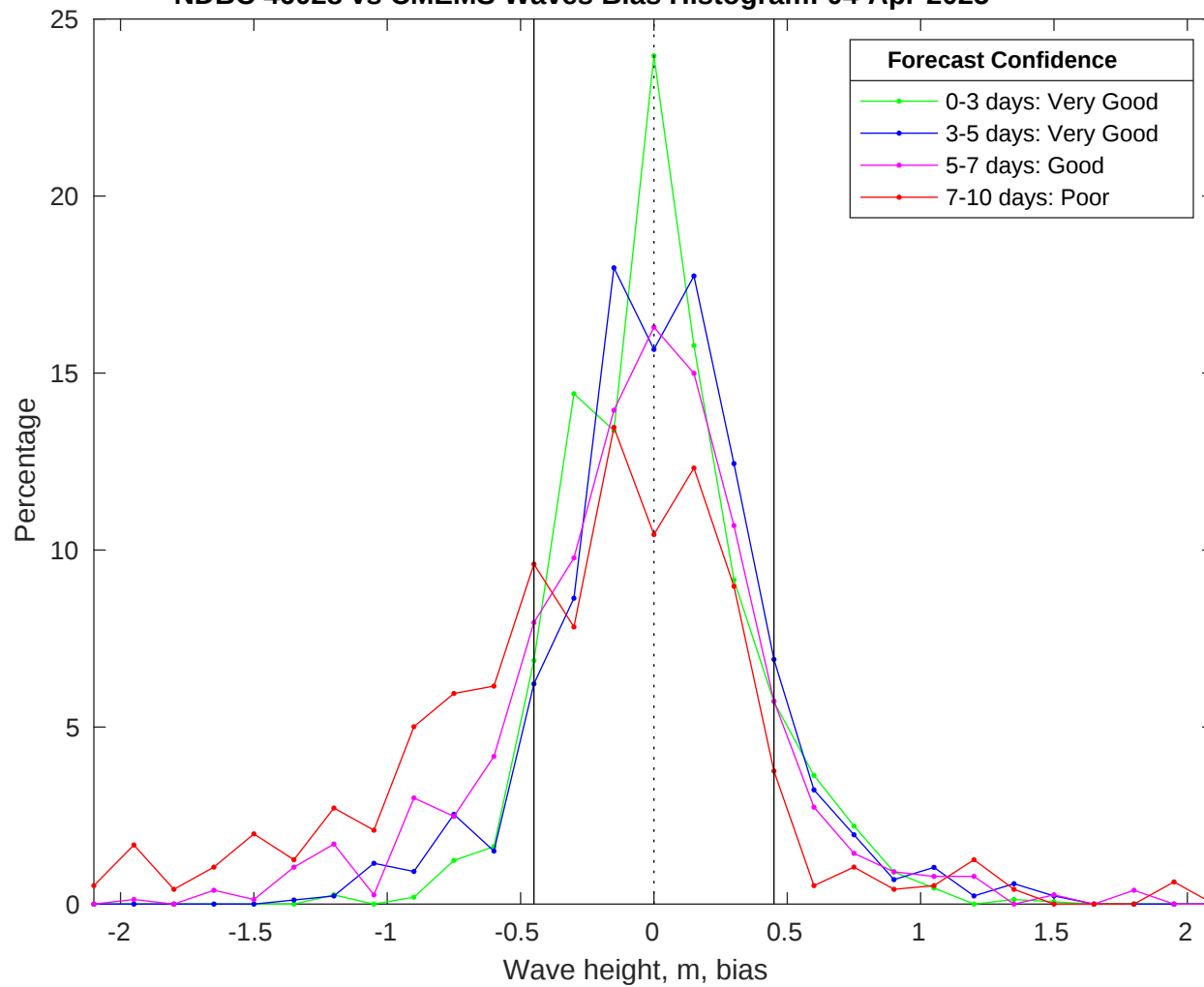
NDBC 46028 vs CMEMS Waves Bias Histogram: 04-Apr-2025
