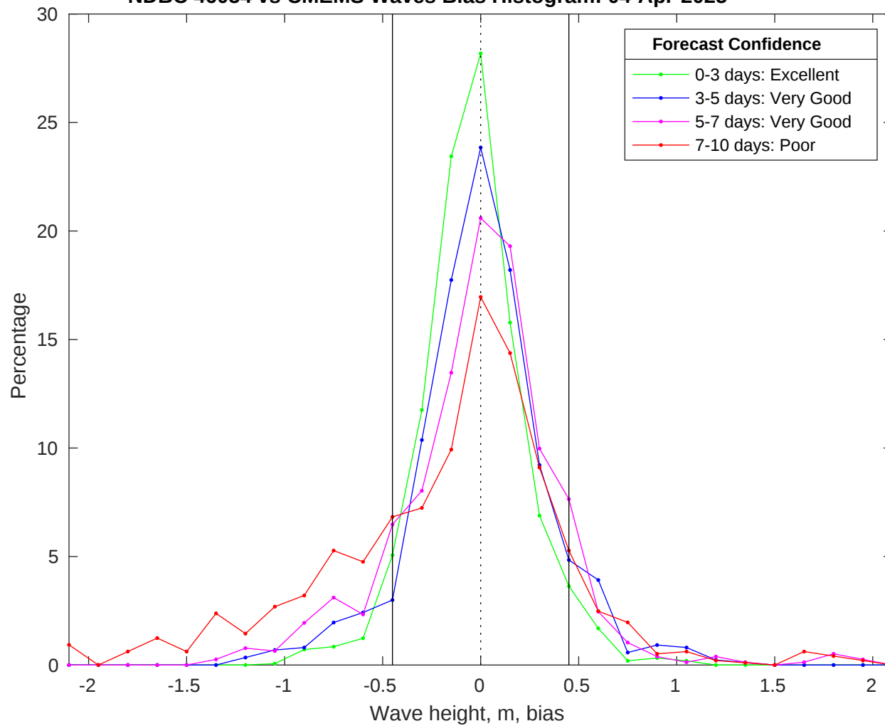
NDBC 46054 vs CMEMS Waves Bias Histogram: 04-Apr-2025
