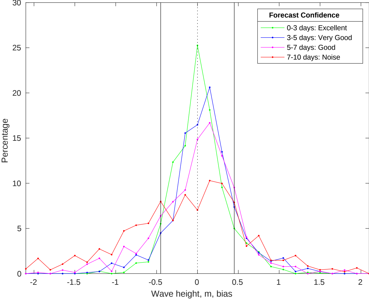
NDBC 46028 vs CMEMS Waves Bias Histogram: 07-Apr-2025
