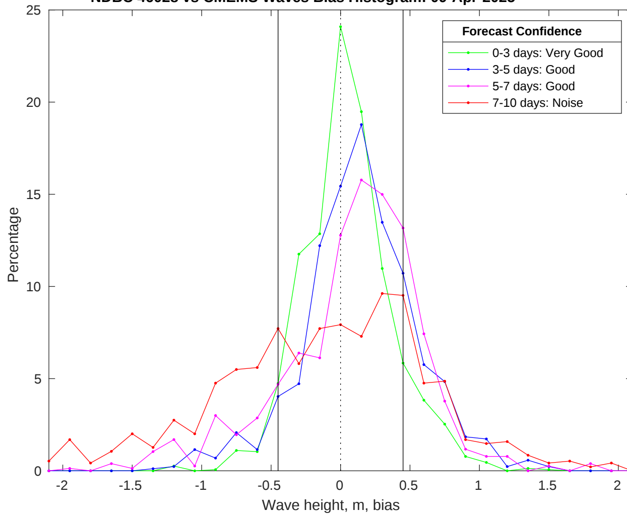
NDBC 46028 vs CMEMS Waves Bias Histogram: 09-Apr-2025
