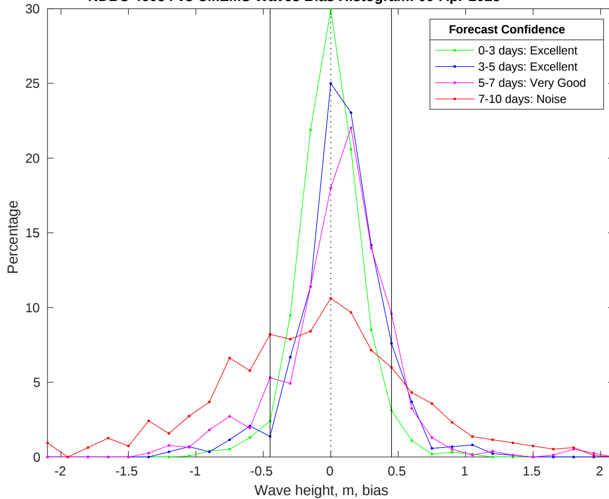
NDBC 46054 vs CMEMS Waves Bias Histogram: 09-Apr-2025
