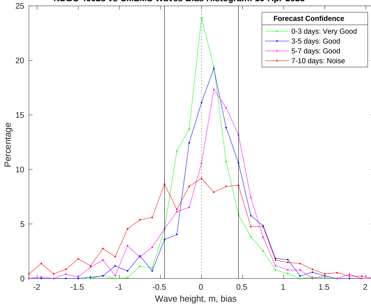
NDBC 46028 vs CMEMS Waves Bias Histogram: 10-Apr-2025
