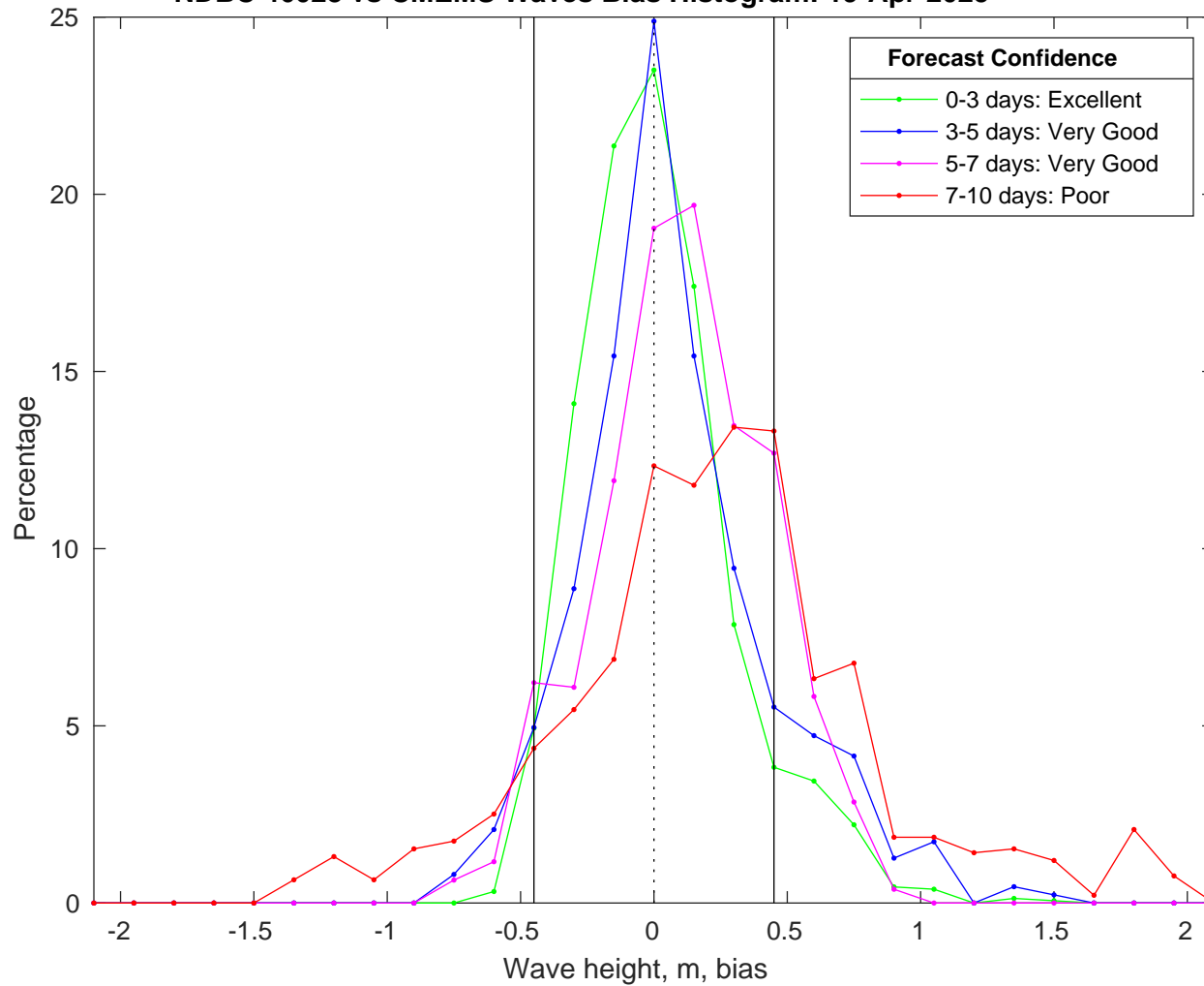
NDBC 46028 vs CMEMS Waves Bias Histogram: 19-Apr-2025
