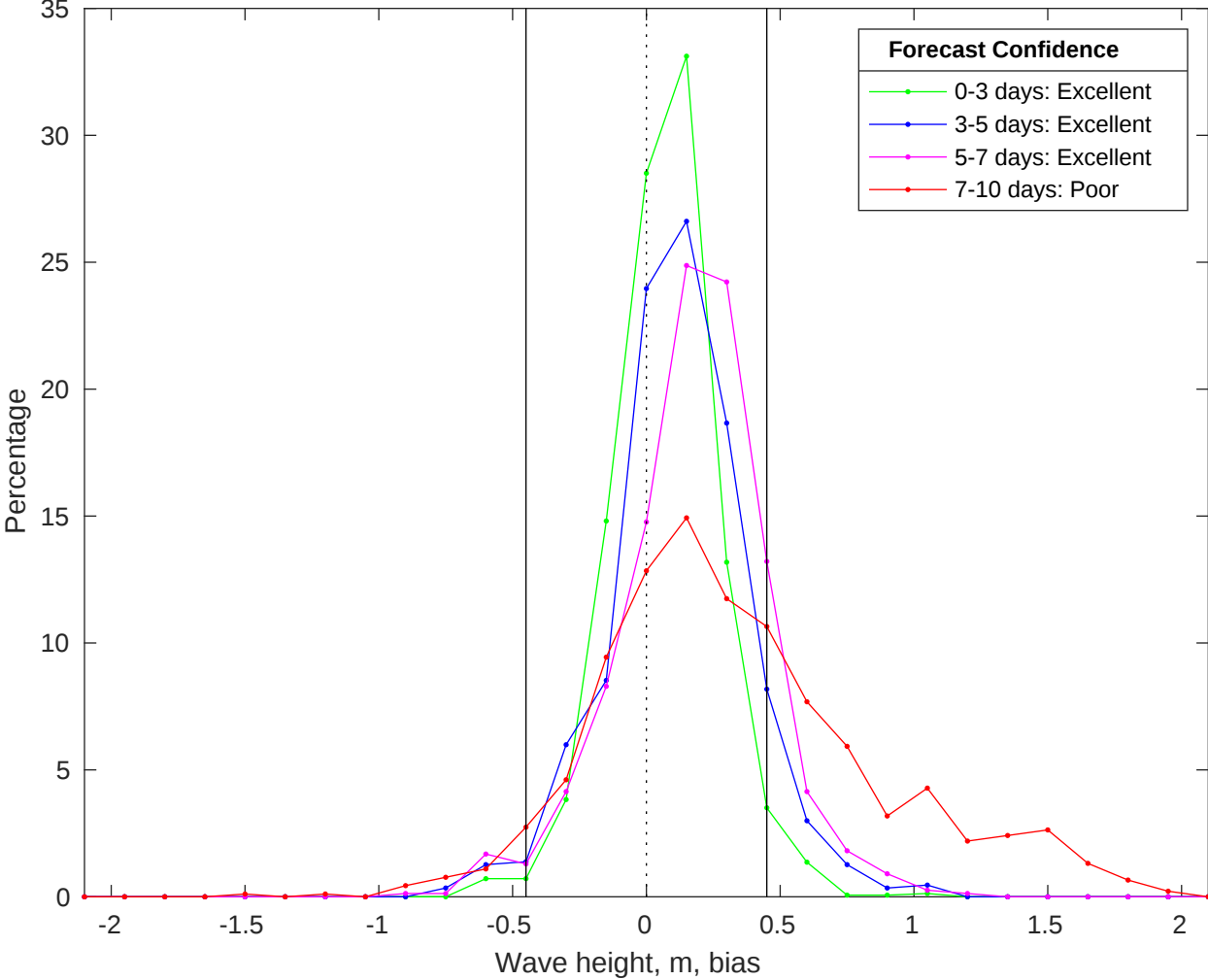
NDBC 46054 vs CMEMS Waves Bias Histogram: 19-Apr-2025
