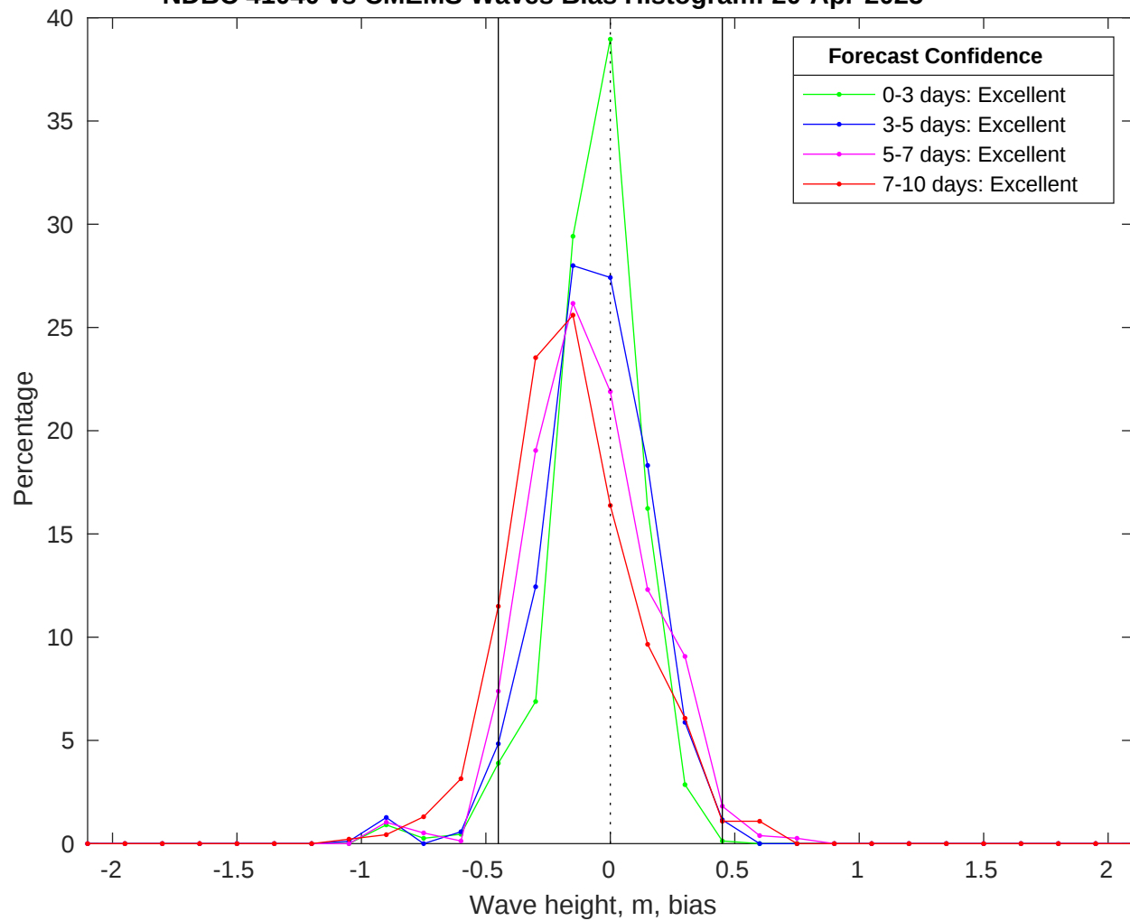
NDBC 41040 vs CMEMS Waves Bias Histogram: 20-Apr-2025
