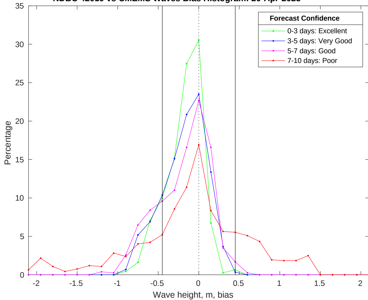
NDBC 42019 vs CMEMS Waves Bias Histogram: 20-Apr-2025
