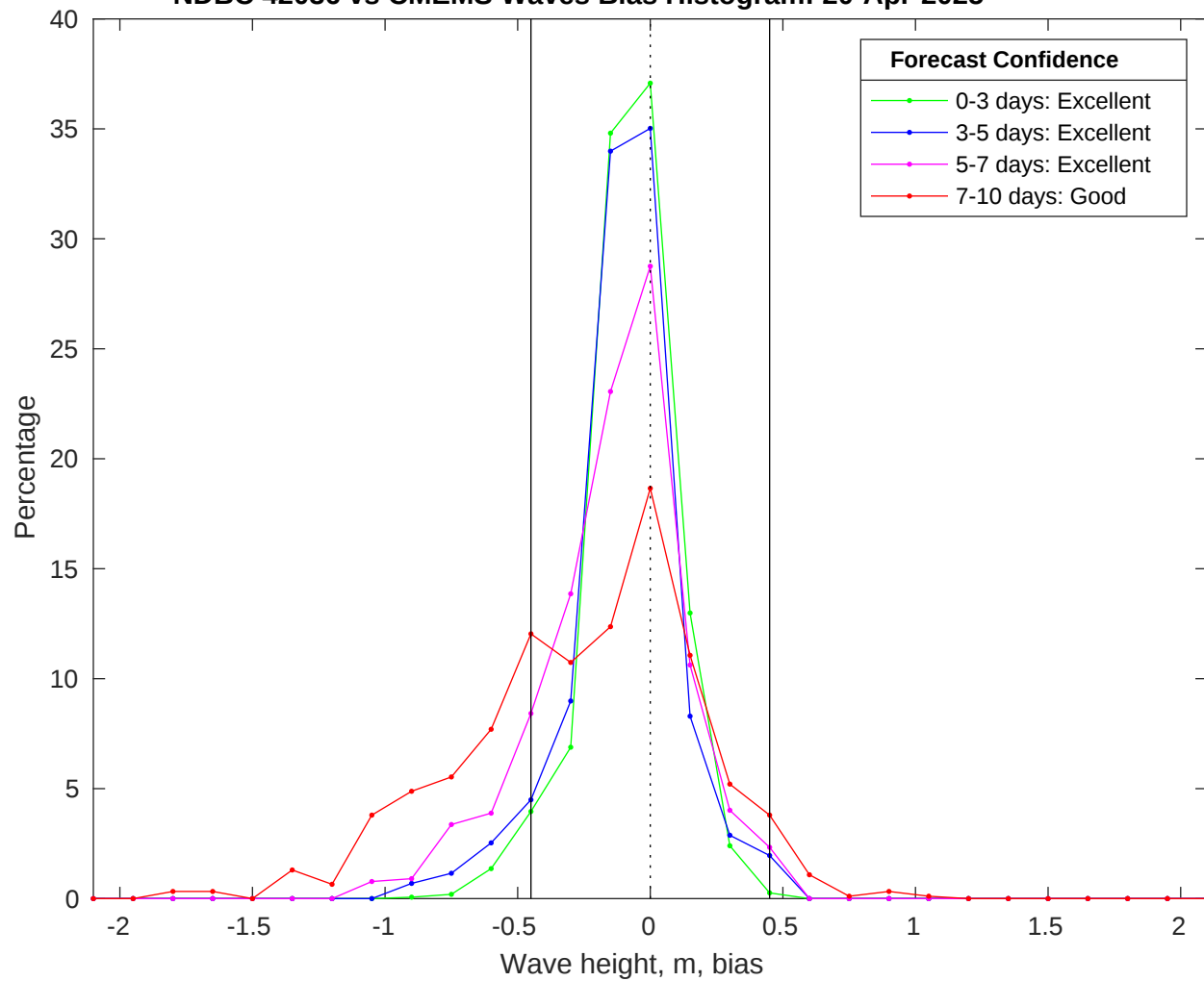
NDBC 42036 vs CMEMS Waves Bias Histogram: 20-Apr-2025
