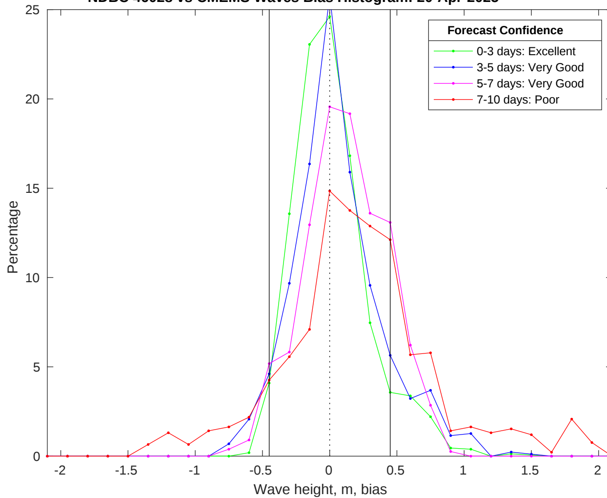
NDBC 46028 vs CMEMS Waves Bias Histogram: 20-Apr-2025
