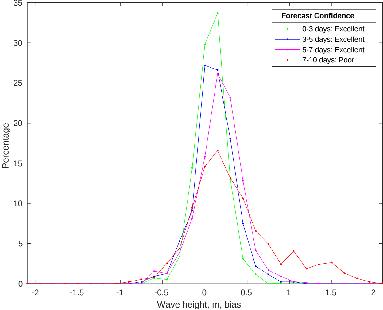
NDBC 46054 vs CMEMS Waves Bias Histogram: 20-Apr-2025
