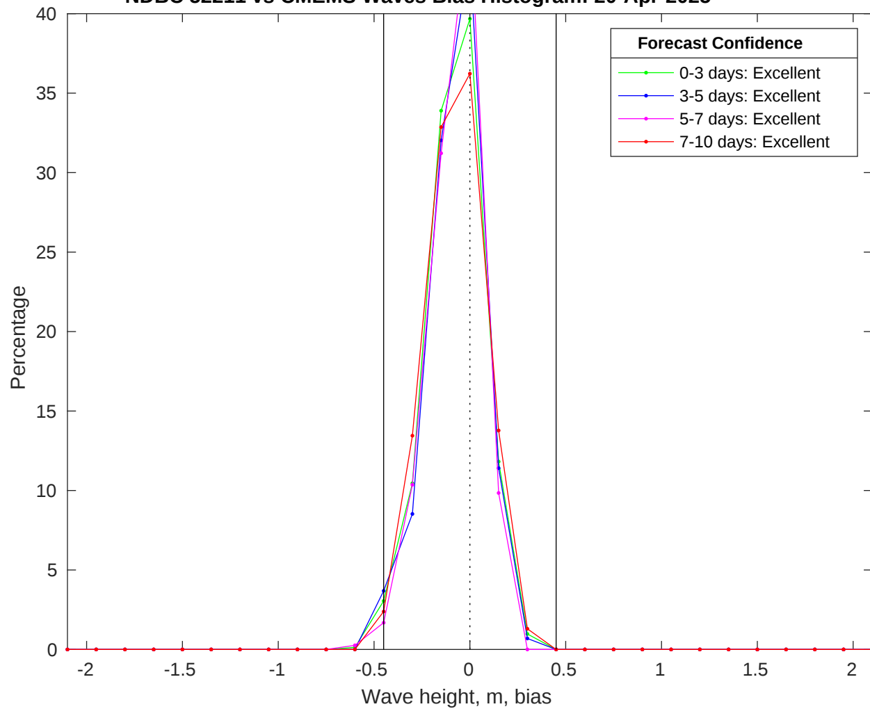
NDBC 52211 vs CMEMS Waves Bias Histogram: 20-Apr-2025
