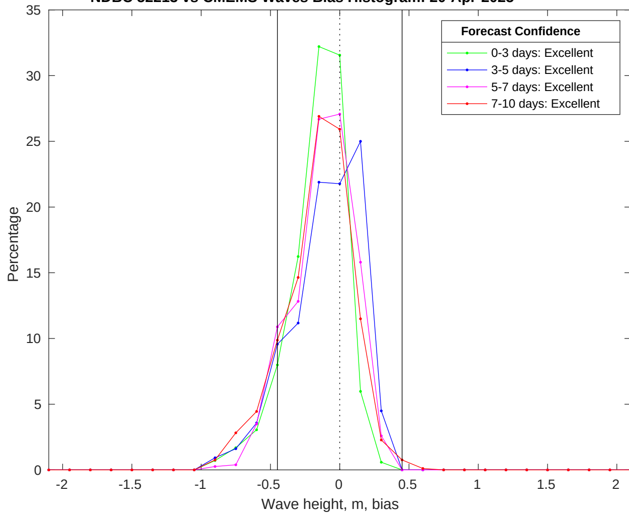
NDBC 52213 vs CMEMS Waves Bias Histogram: 20-Apr-2025
