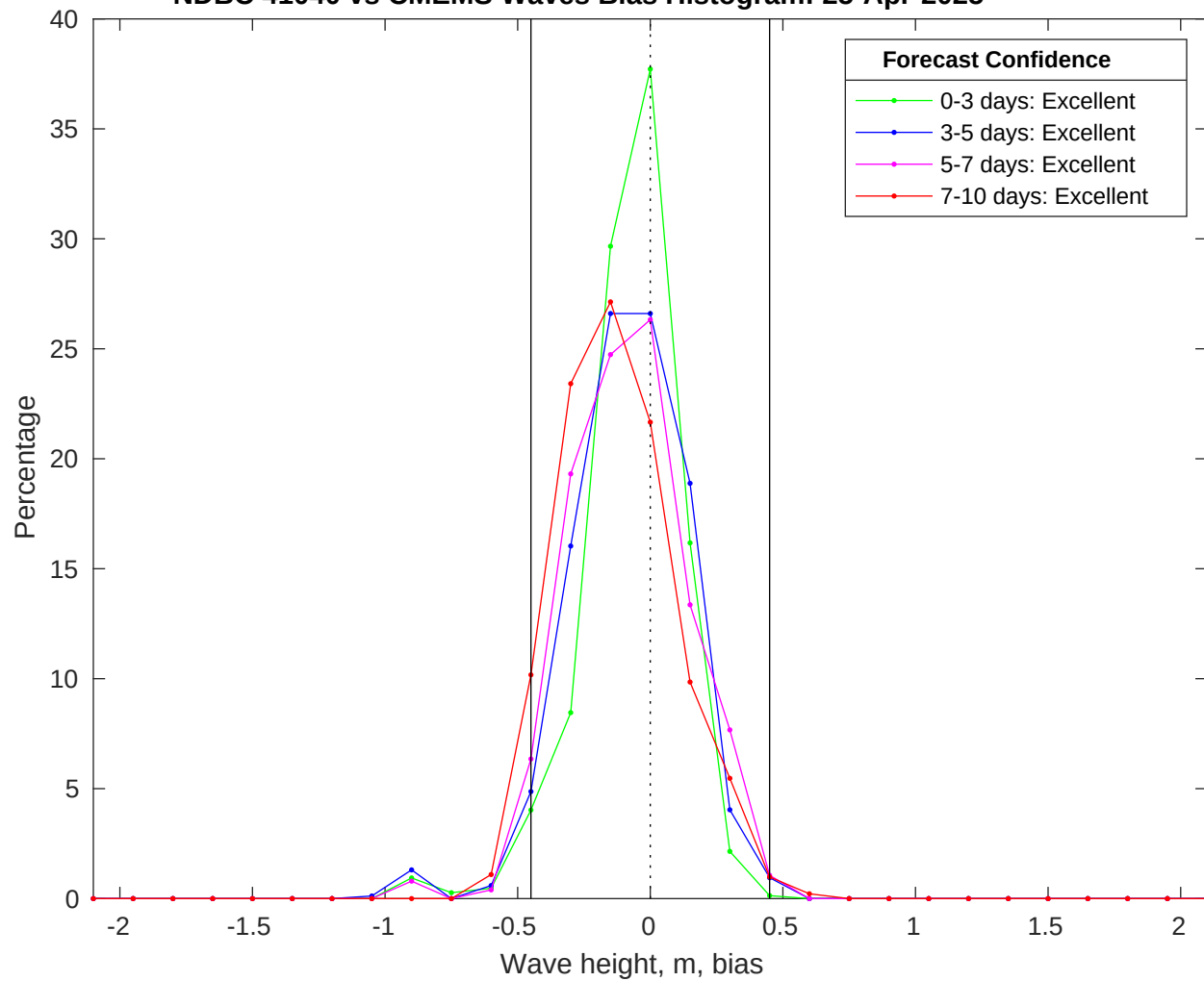
NDBC 41040 vs CMEMS Waves Bias Histogram: 25-Apr-2025
