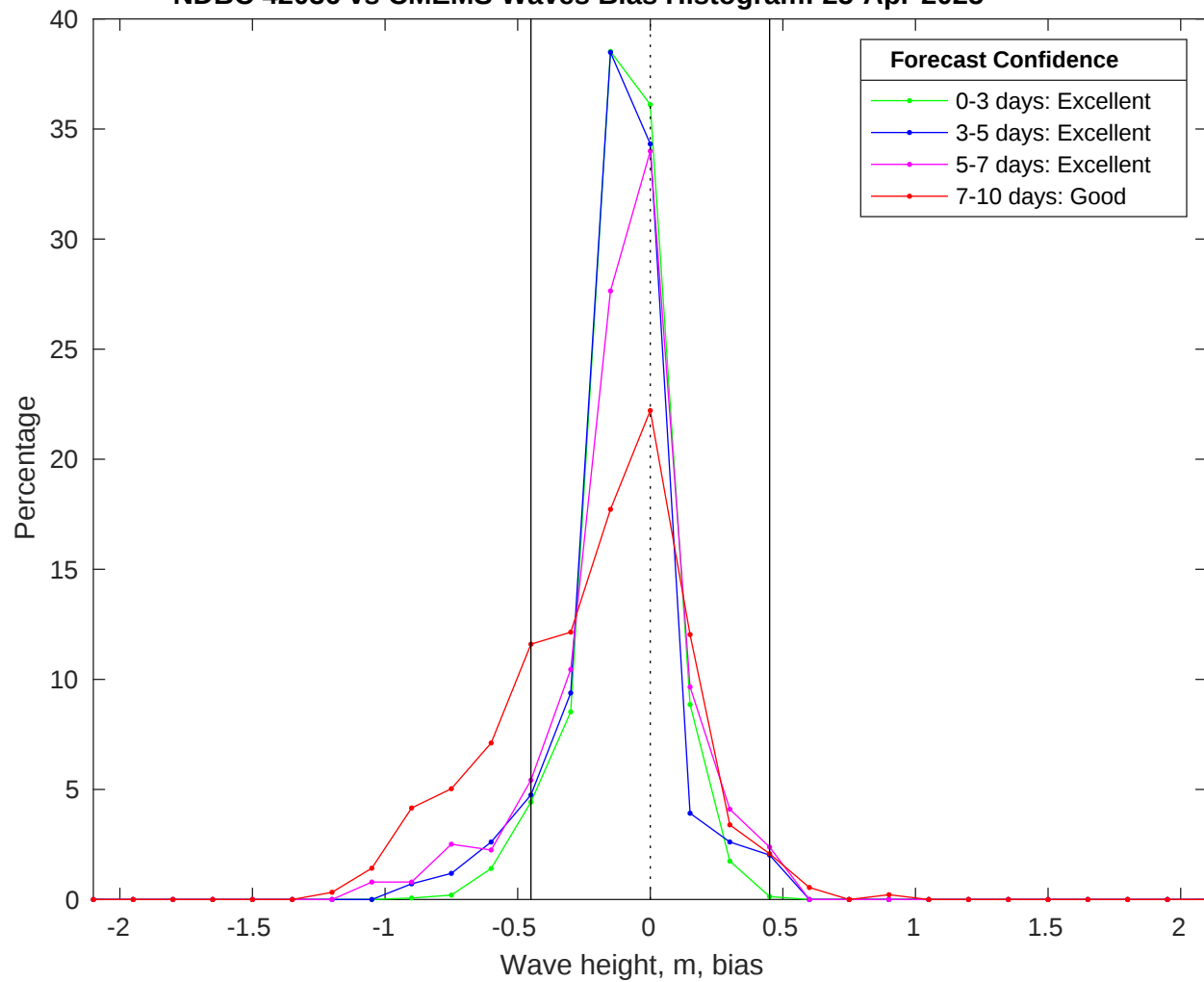
NDBC 42036 vs CMEMS Waves Bias Histogram: 25-Apr-2025
