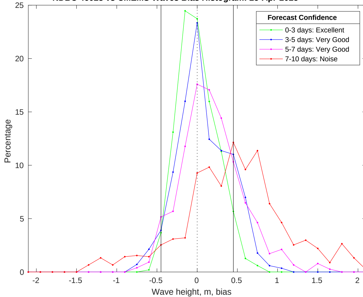
NDBC 46028 vs CMEMS Waves Bias Histogram: 25-Apr-2025
