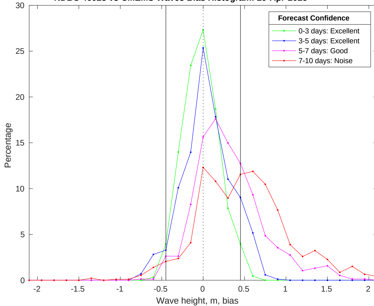
NDBC 46028 vs CMEMS Waves Bias Histogram: 29-Apr-2025
