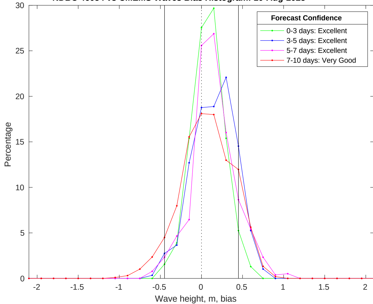
NDBC 46054 vs CMEMS Waves Bias Histogram: 10-Aug-2025
