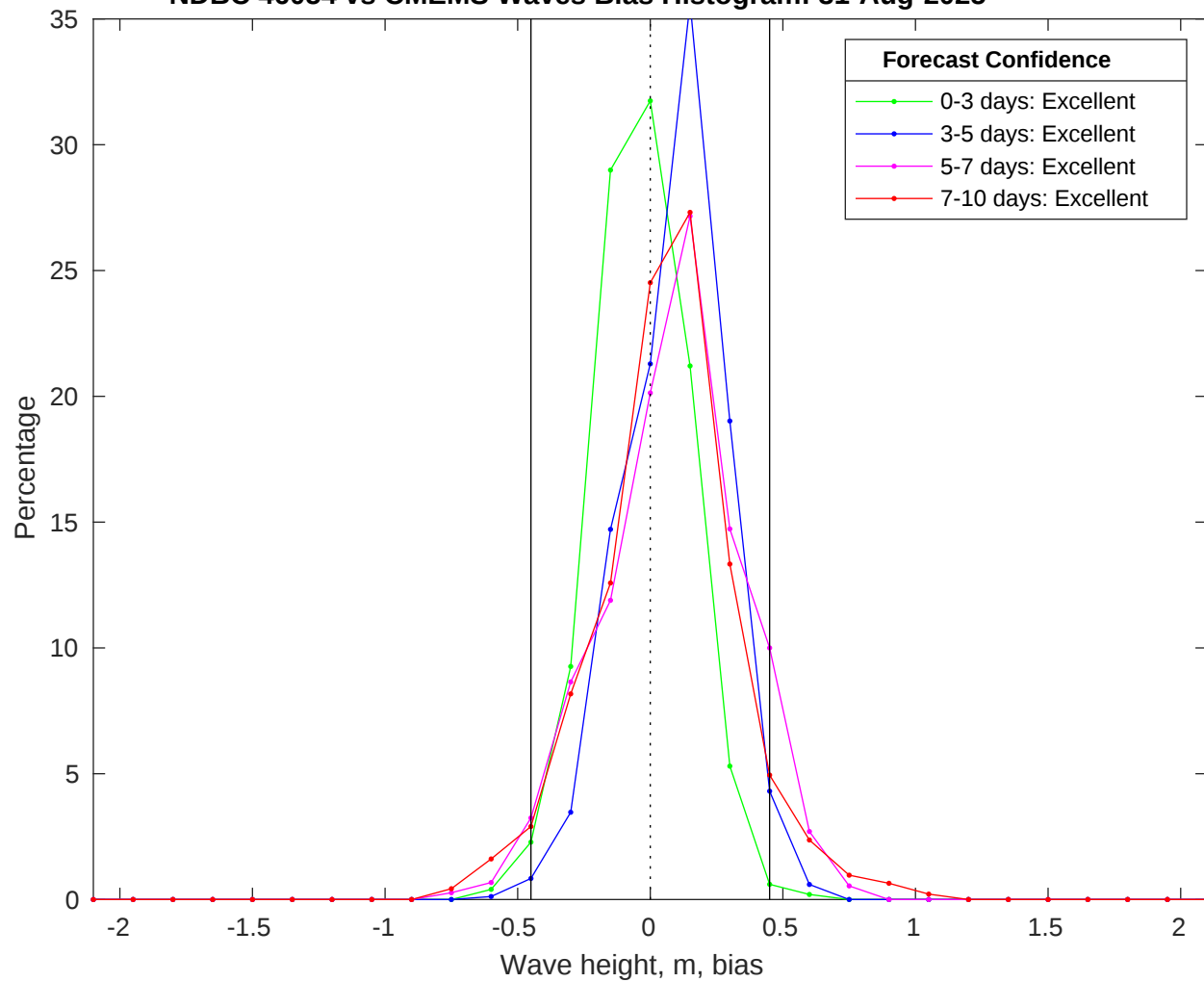
NDBC 46054 vs CMEMS Waves Bias Histogram: 31-Aug-2025
