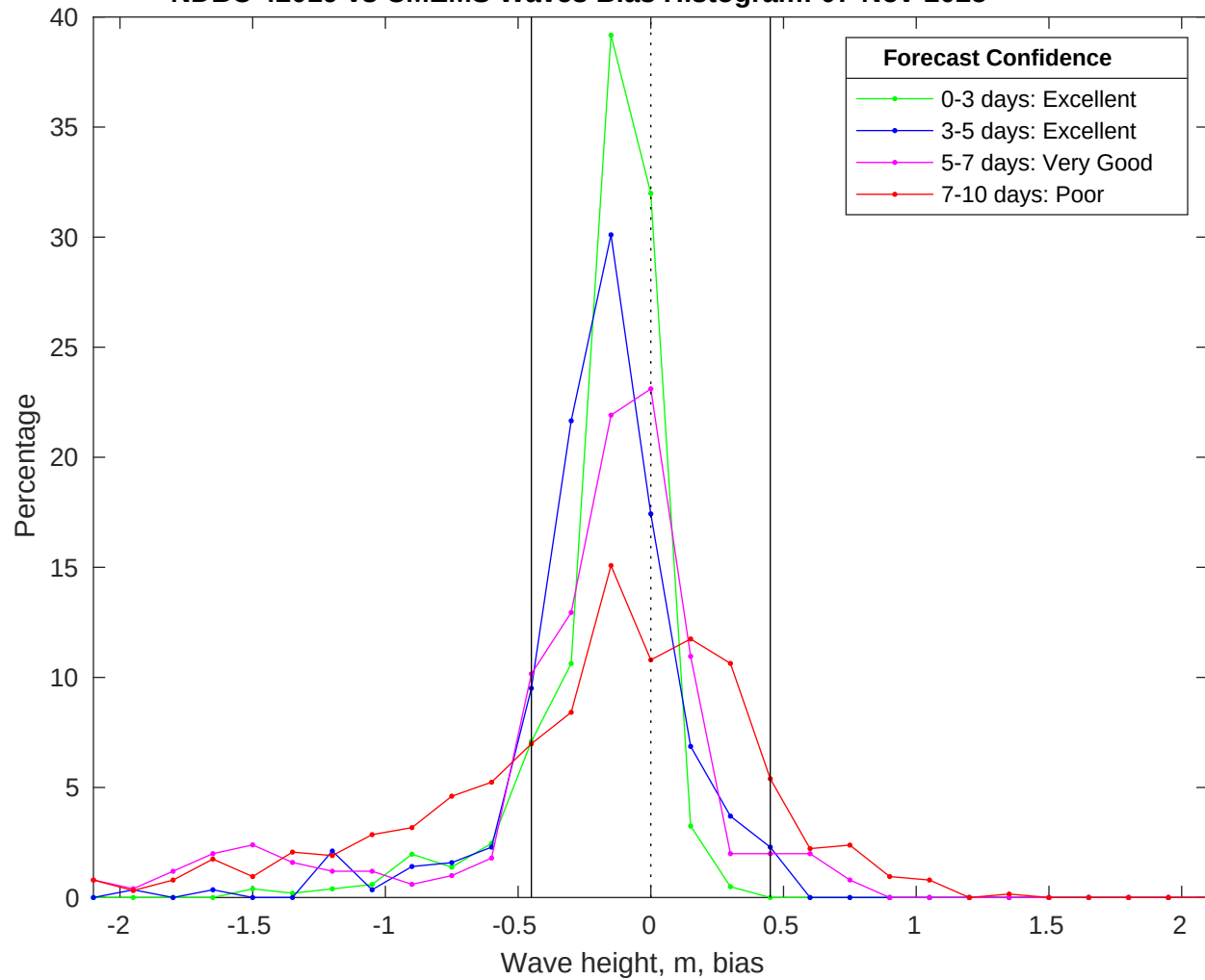
NDBC 42019 vs CMEMS Waves Bias Histogram: 07-Nov-2025
