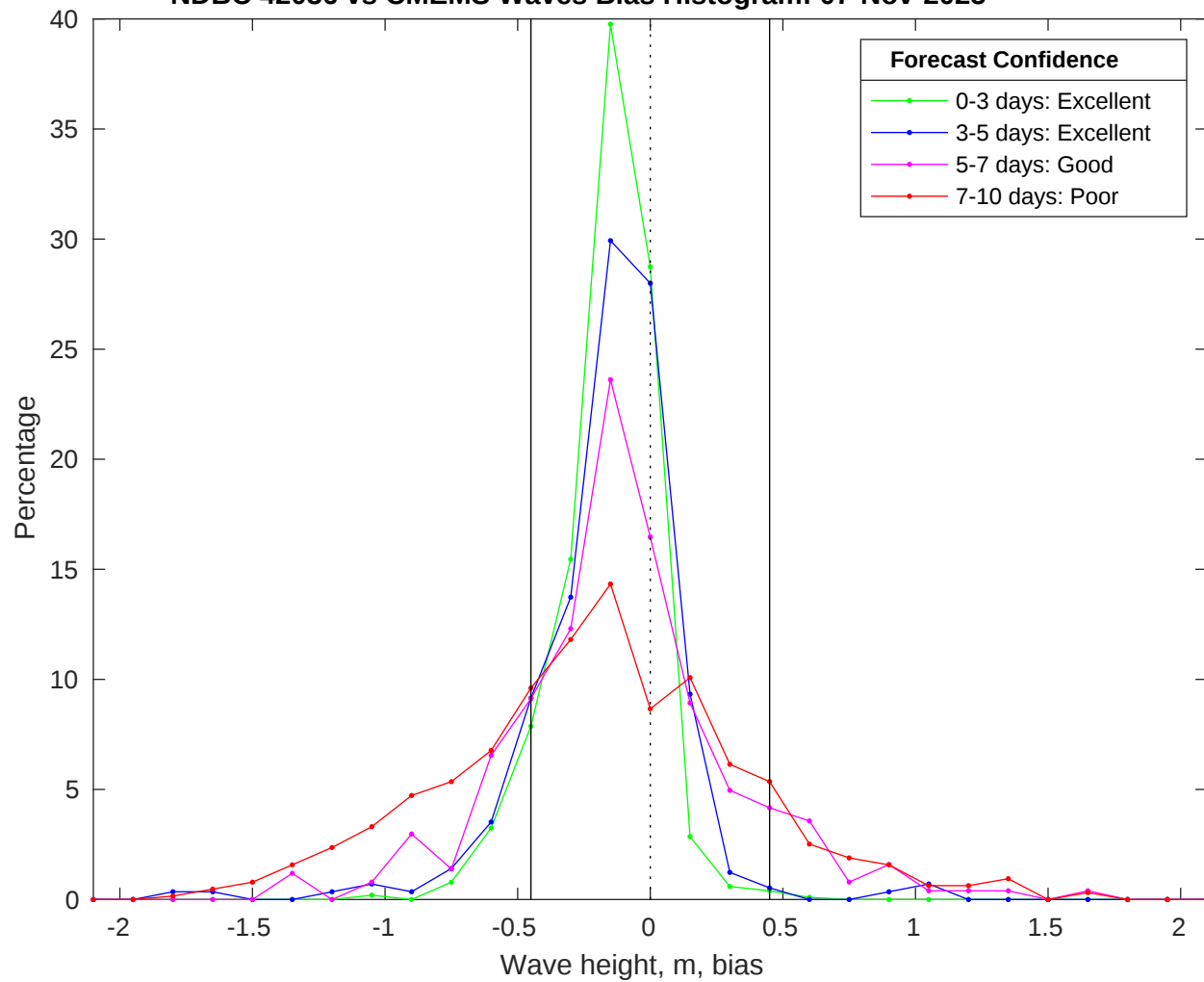
NDBC 42036 vs CMEMS Waves Bias Histogram: 07-Nov-2025
