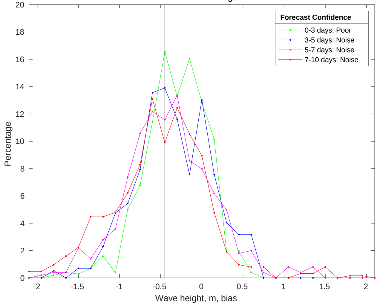
NDBC 46028 vs CMEMS Waves Bias Histogram: 07-Nov-2025
