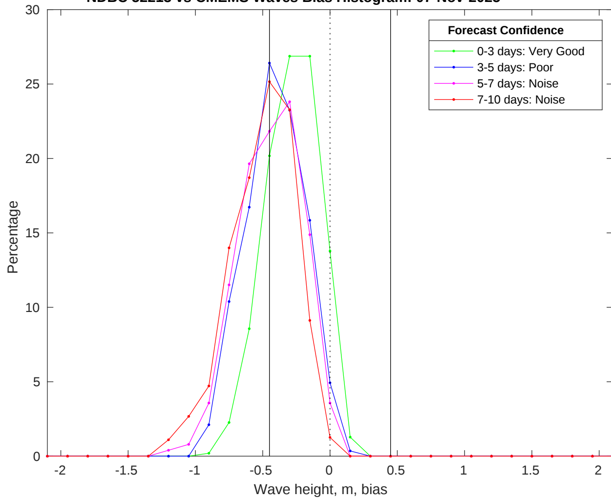
NDBC 52213 vs CMEMS Waves Bias Histogram: 07-Nov-2025
