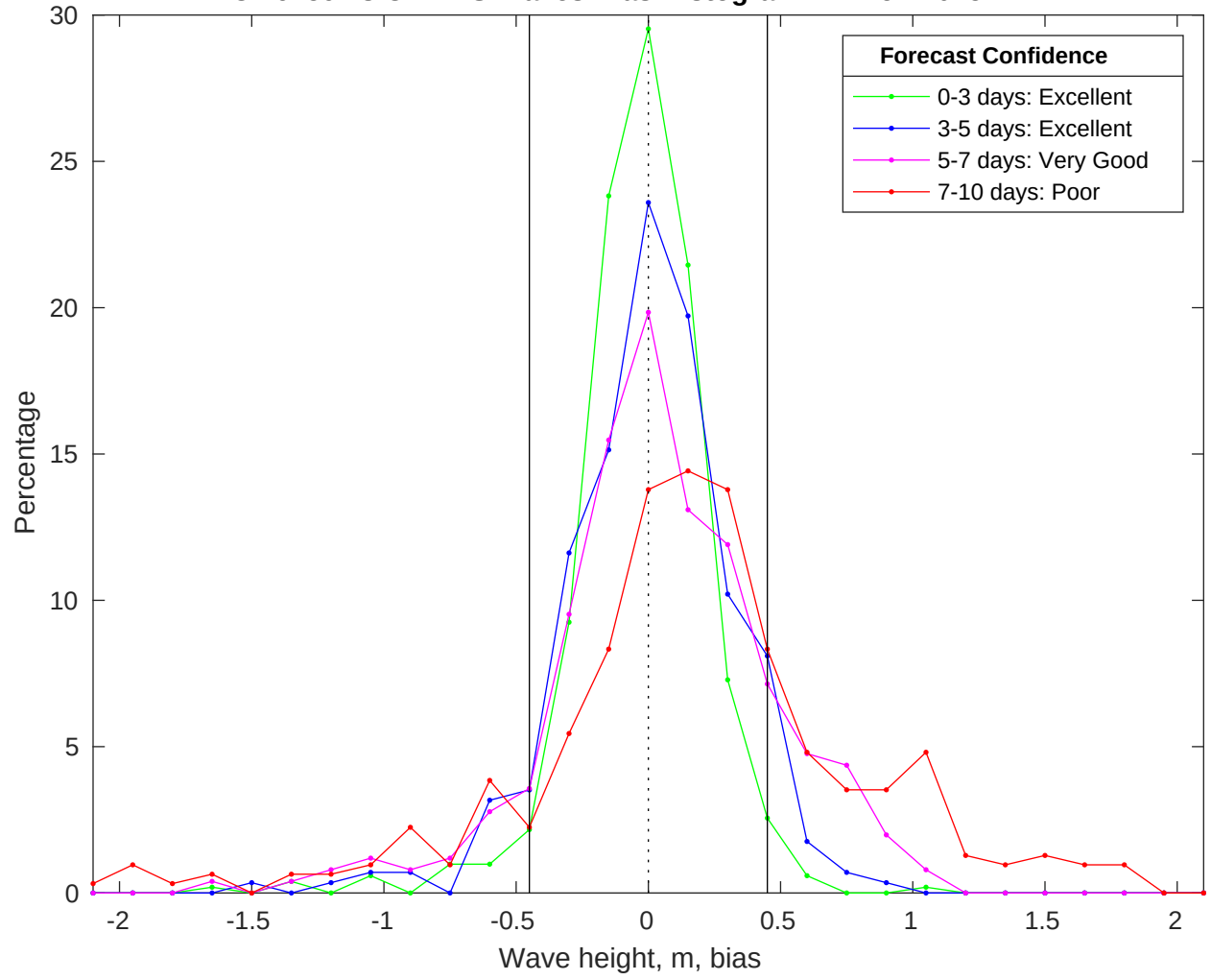
NDBC 46259 vs CMEMS Waves Bias Histogram: 17-Nov-2025
