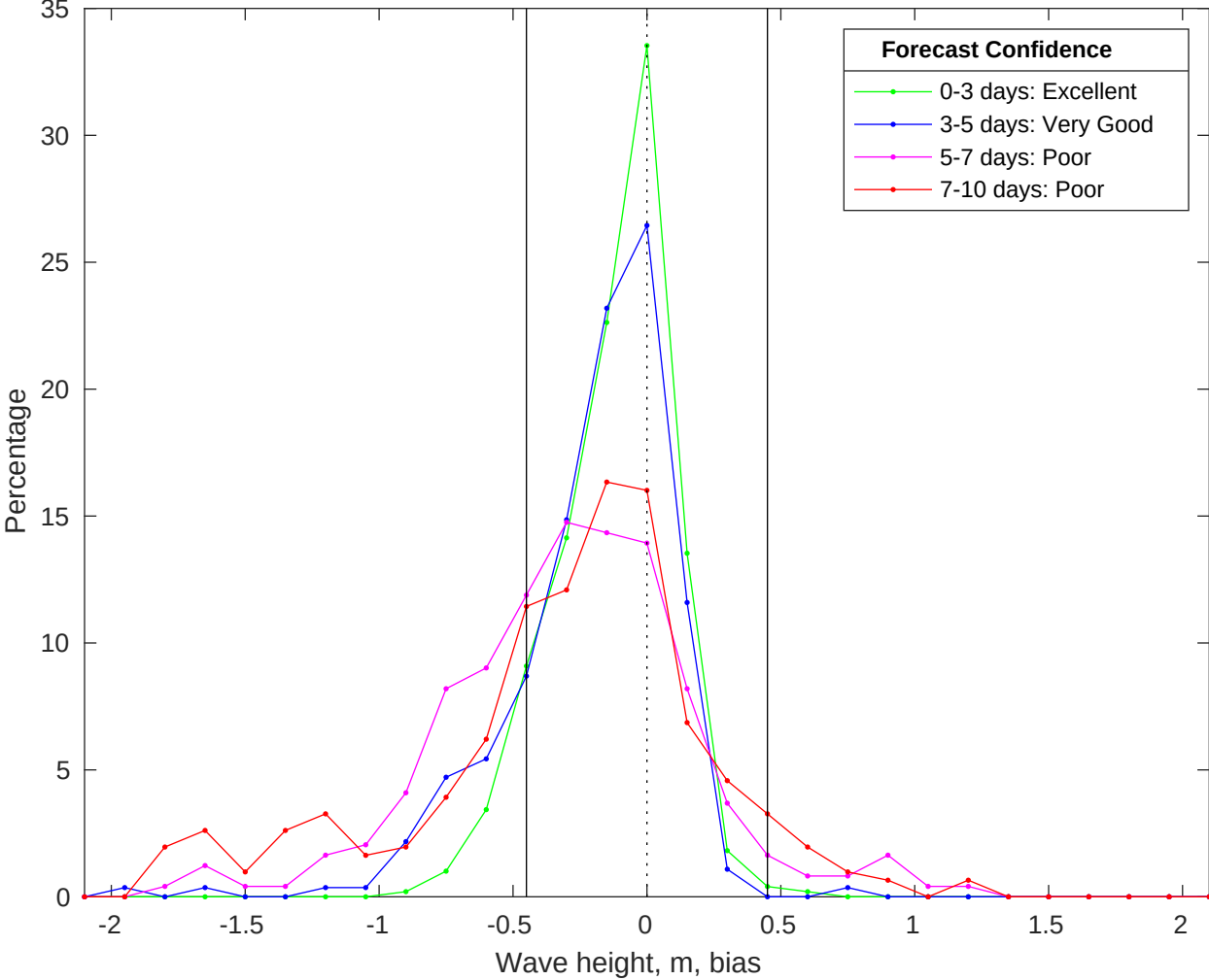
NDBC 41013 vs CMEMS Waves Bias Histogram: 02-Jan-2026
