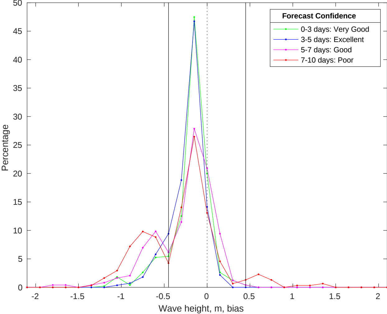
NDBC 42036 vs CMEMS Waves Bias Histogram: 02-Jan-2026
