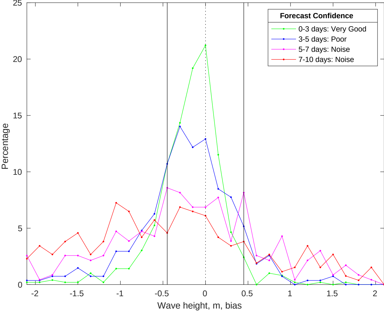
NDBC 44008 vs CMEMS Waves Bias Histogram: 02-Jan-2026
